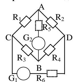
Рис.2.2.Схема моста
