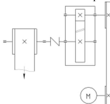
Кинематическая схема привода
