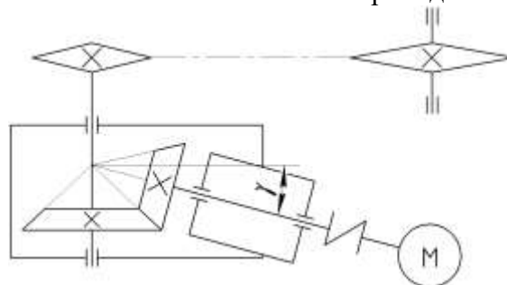
Кинематическая схема привода
