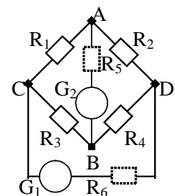
Рис.2.2.Схема моста
