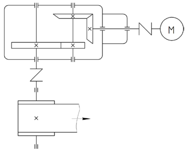
Кинематическая схема привода
