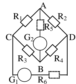
Рис.2.2.Схема моста
