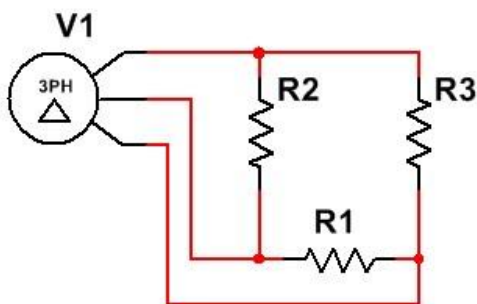
Рис. 9. Схема трехфазной цепи при соединении нагрузки треугольником
